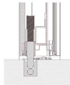
Sezione inferiore con Kit soglia
