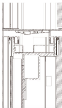
Sezione superiore con Kit soglia
