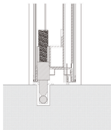
Sezione inferiore con antispiffero
