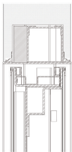
Sezione superiore con antispiffero
